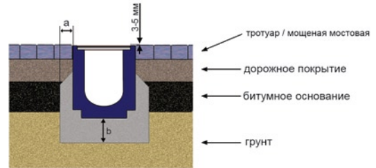
Рис. 1.1. - Схема по установке каналов
