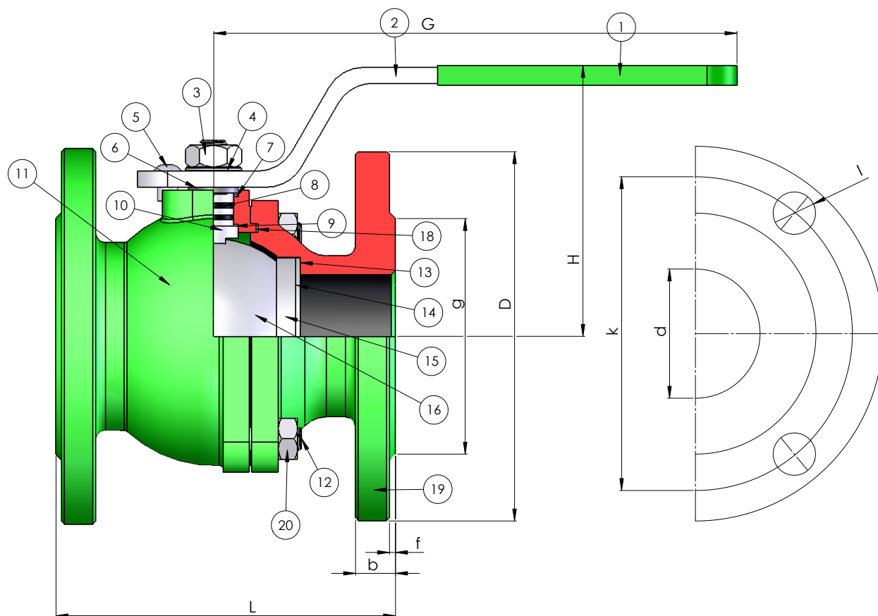
FAF 1220 КРАН ШАРОВОЙ ФЛАНЦЕВЫЙ Ру 16
